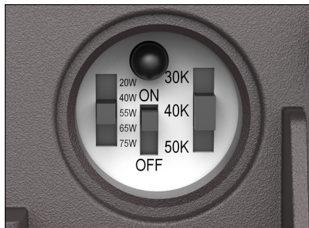
Sélecteurs de puissance, TCC et photocellule
